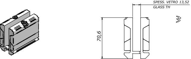
Set pinze di fissaggio Sirio Small Sirio Small clamping set
