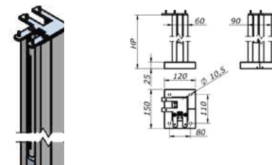
Piastra di fissaggio a 90° per corrimano 90° fixing plate for handrail
