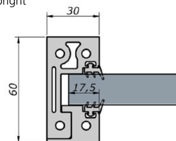
Montante terminale Lateral upright
