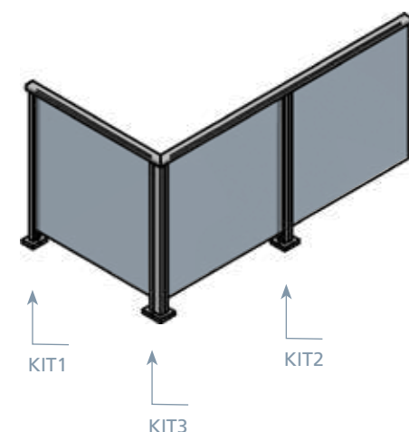
Montante tutta altezza con profilo corrimano Full height upright with handrail profile
