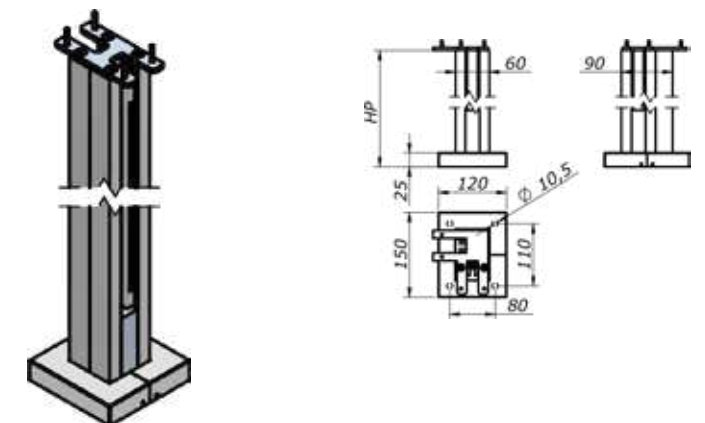
Piastra di fissaggio centrale per corrimano Central fixing plate for handrail
