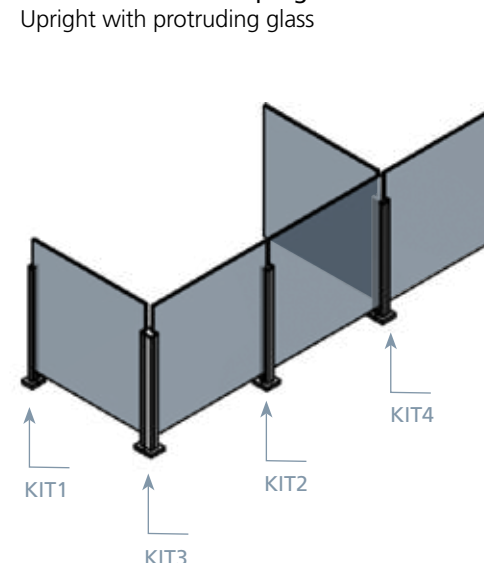
Montante con vetro sporgente Upright with protruding glass
