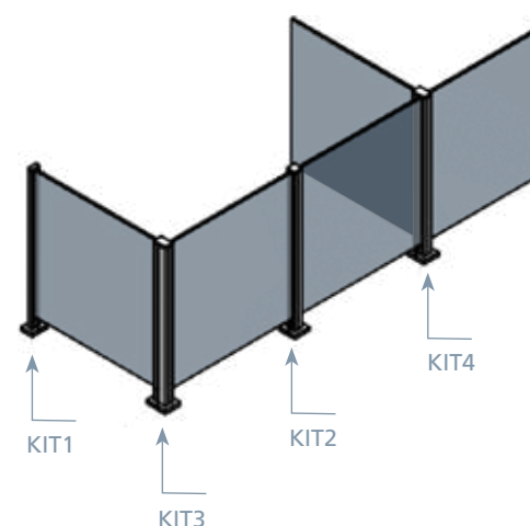
Montante tutta altezza con profilo corrimano Full height upright with handrail profile
