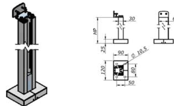
Piastra di fissaggio corrimano laterale incluso tappo Side fixing plate for handrail including lateral cap
