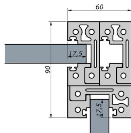
Montante ad angolo a due vie Two-way corner upright
